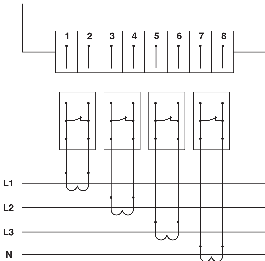
Diagrama eléctrico
