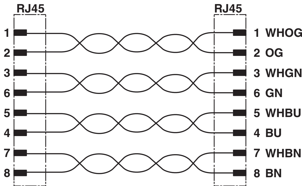
Ocupación de contactos de los conectores macho RJ45
