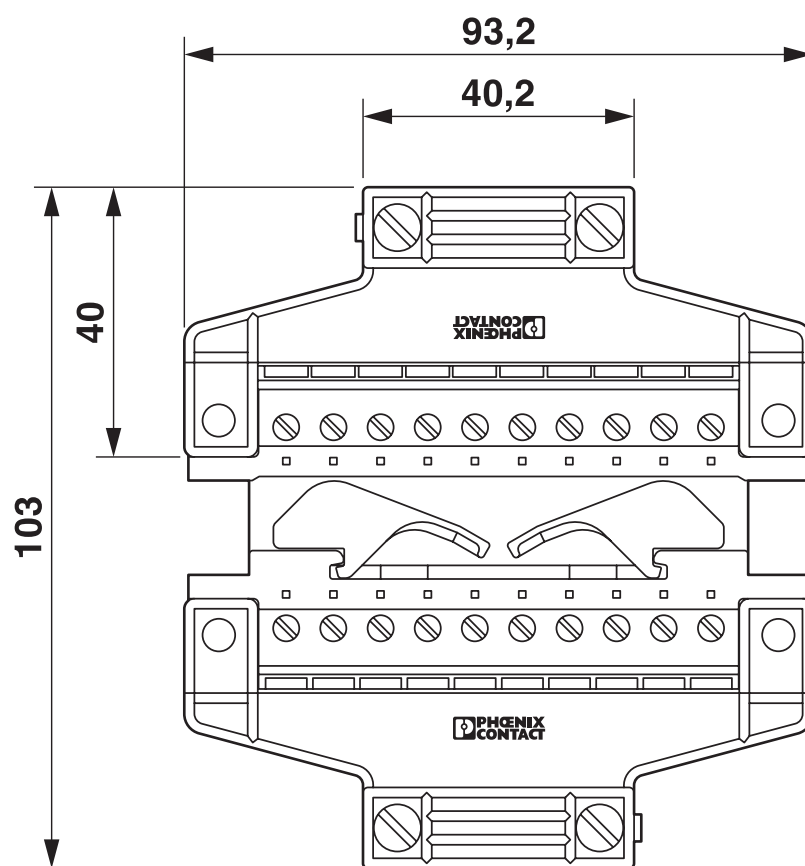
Dessin coté
