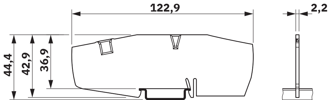
Maßzeichnung
