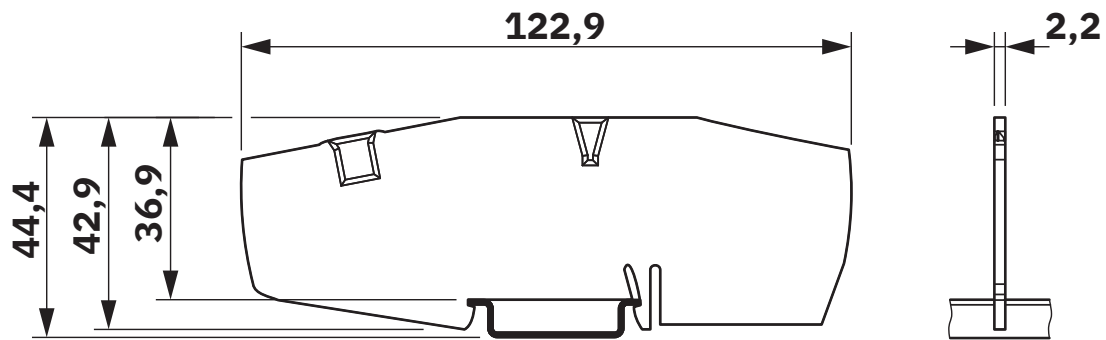
Dessin coté
