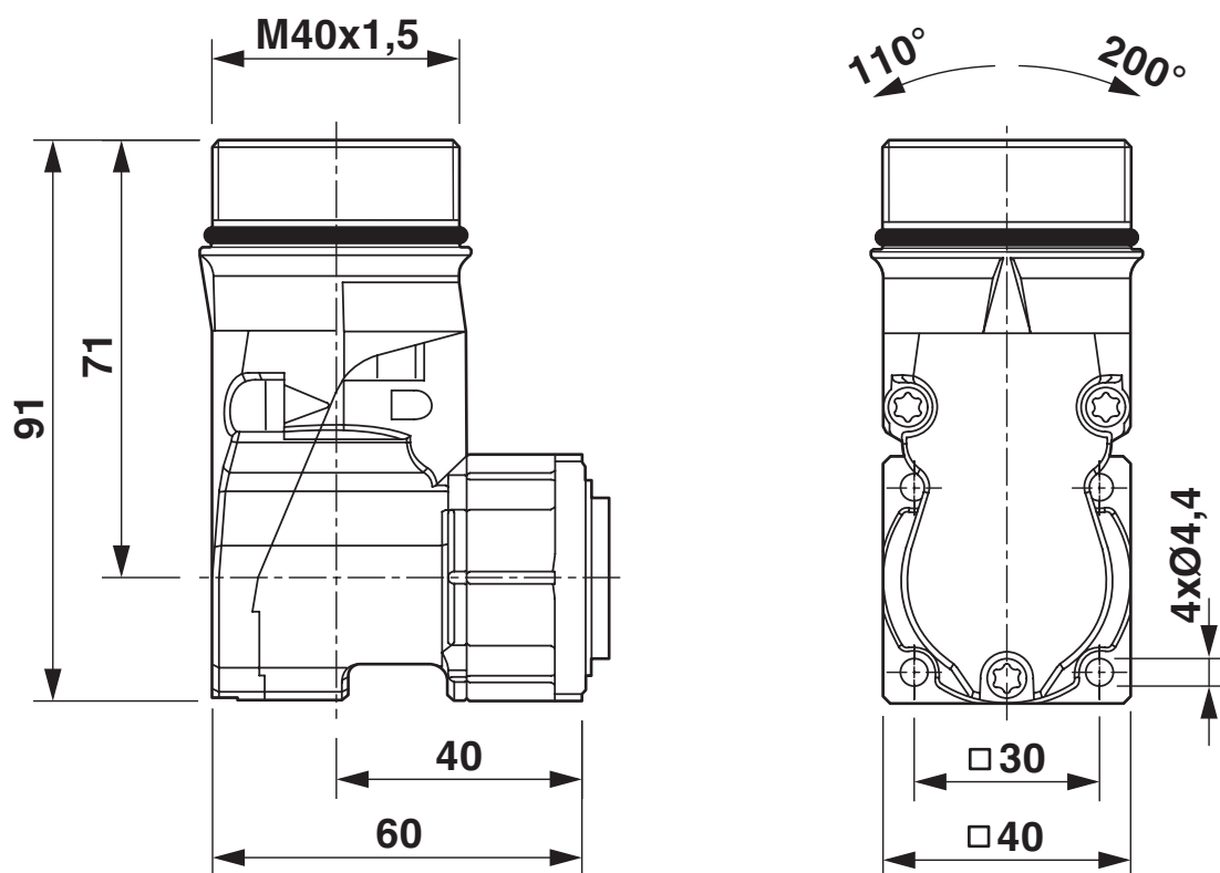
Dessin coté
