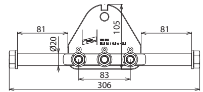
Maßbild PAP 3 M12 SSM B13 RB
