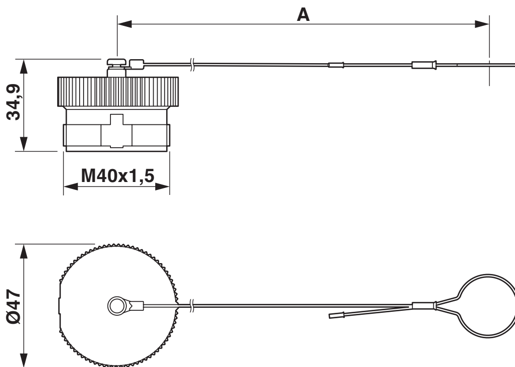
Maßzeichnung
