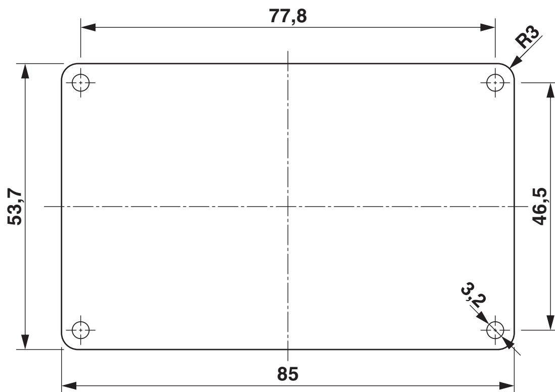
Dessin coté
