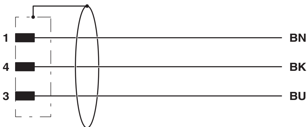
Diagrama eléctrico
