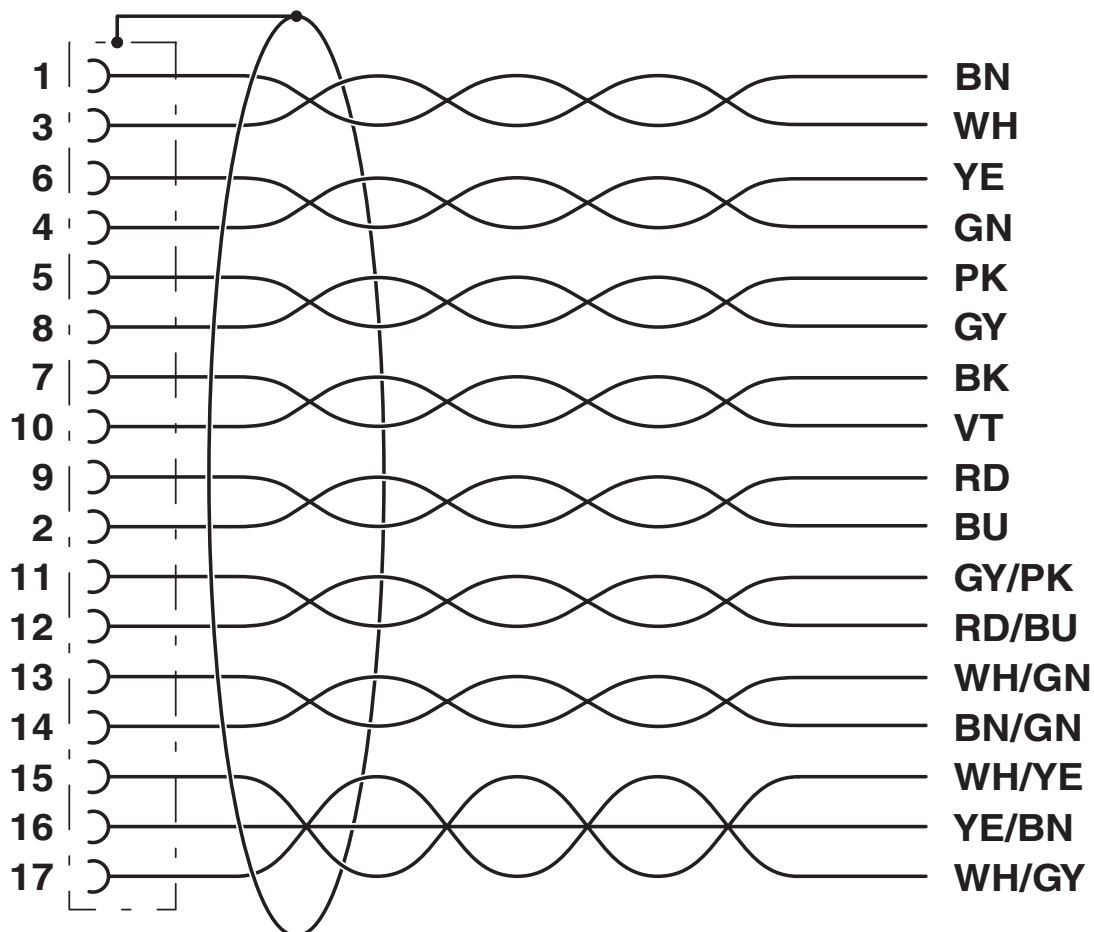
Diagrama eléctrico
