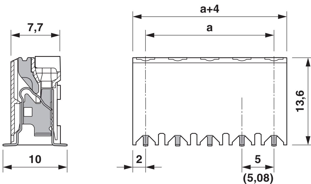
Maßzeichnung
