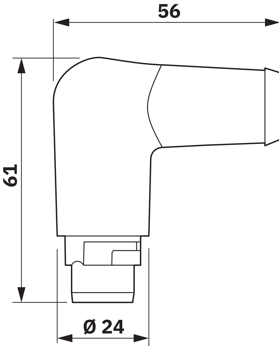
S15-Stecker, gewinkelt
