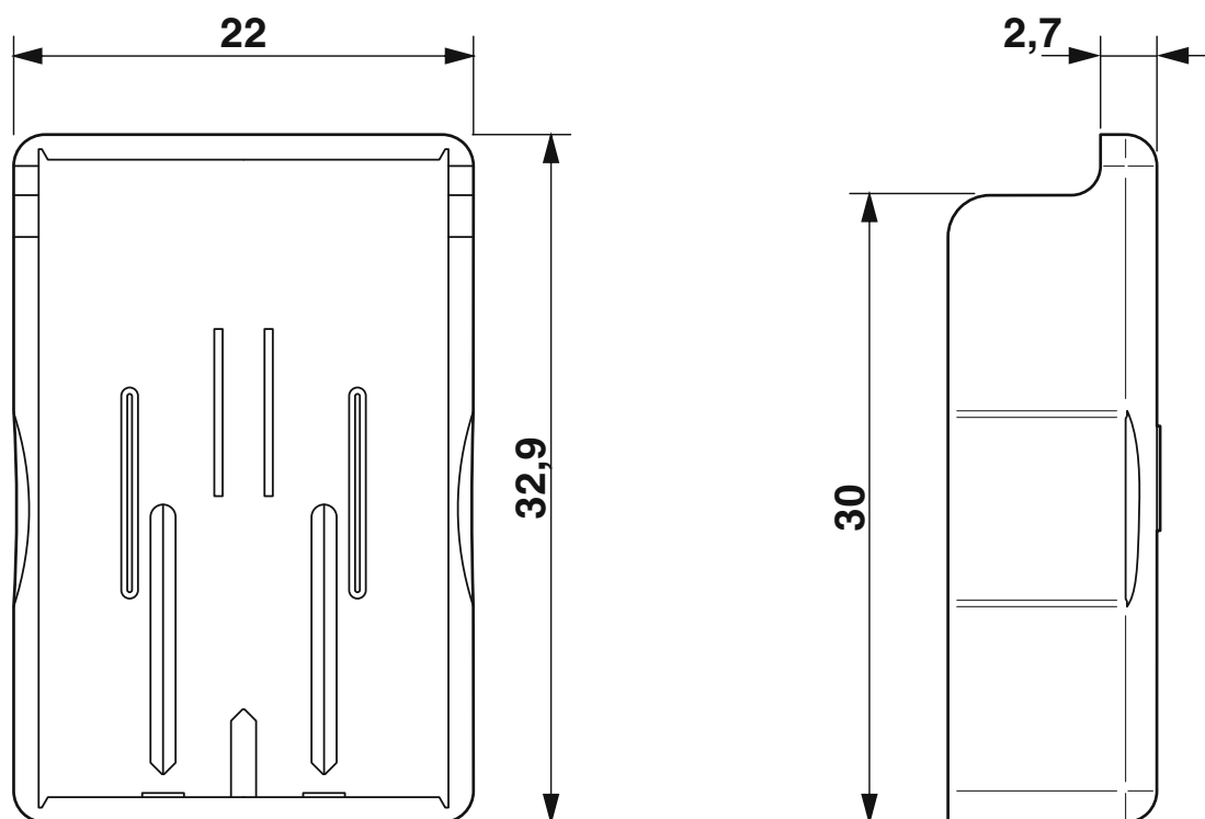
Maßzeichnung
