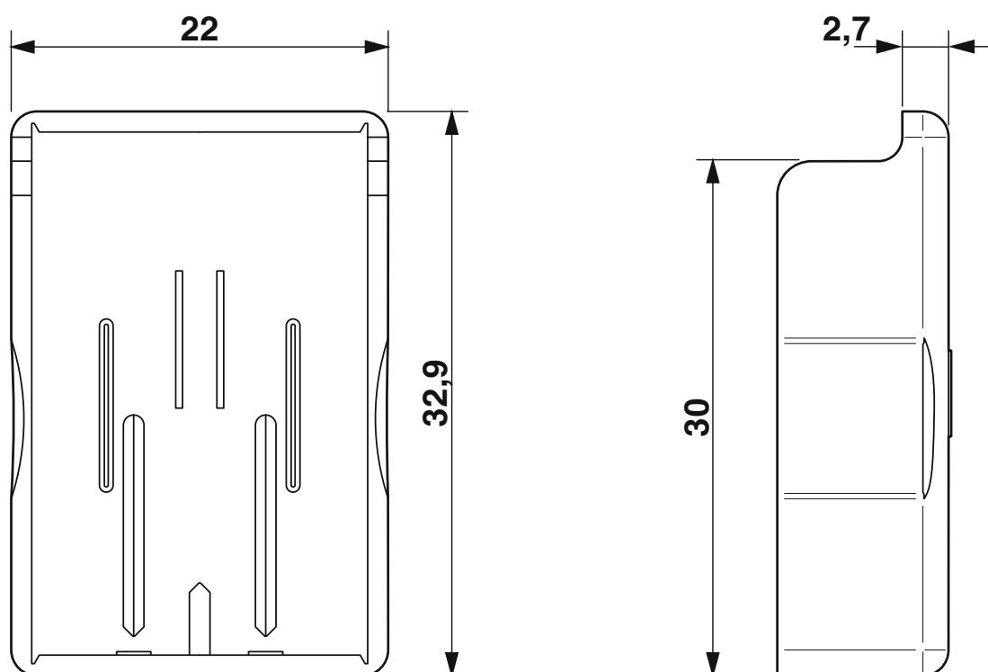
Dessin coté
