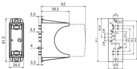
Dimensioni DG PCB PV SCI 600 FM
