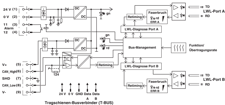
Blockschaltbild
