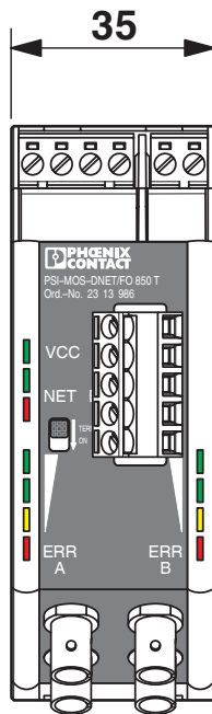
Gehäuseabmessungen
