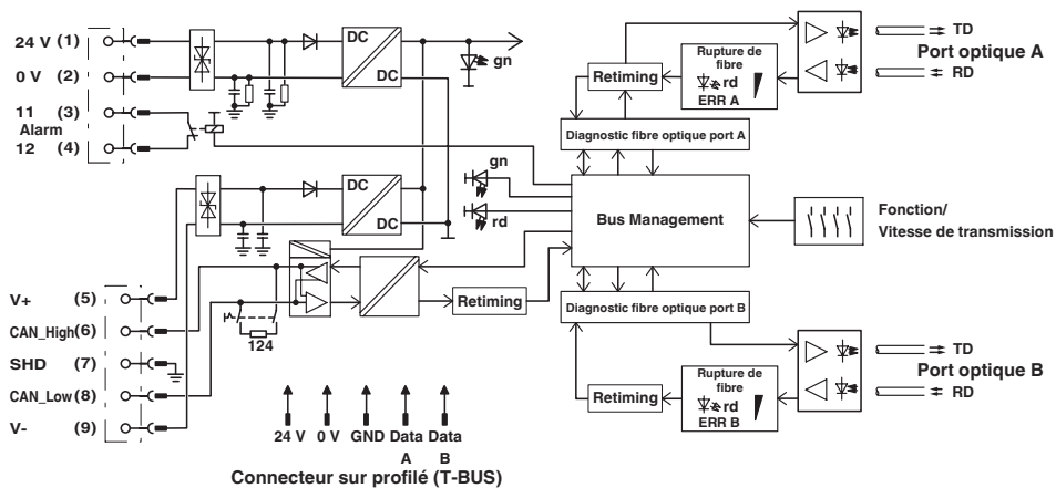
Schéma fonctionnel
