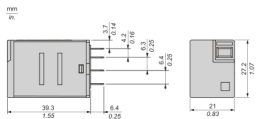
Stecker-Seitenansicht
