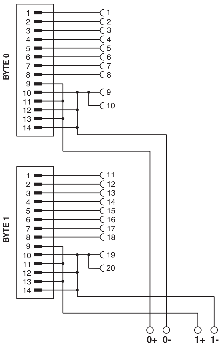
Schaltplan
