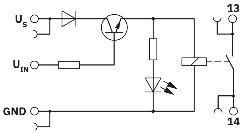
Schéma de connexion
