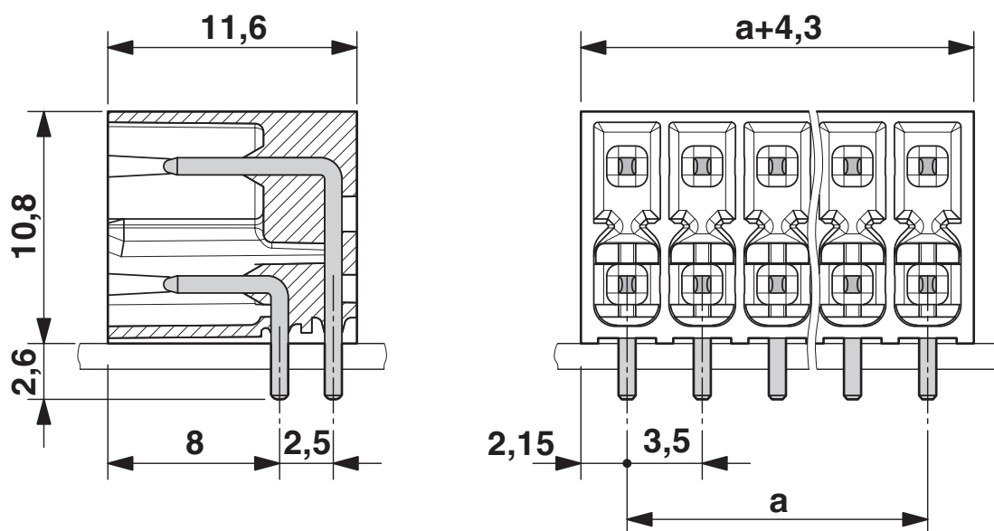
Dessin schématique
