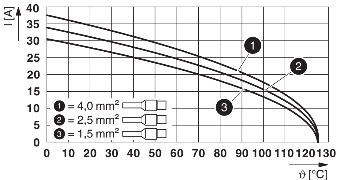
Diagrama de derating (en estado desenchufado)
