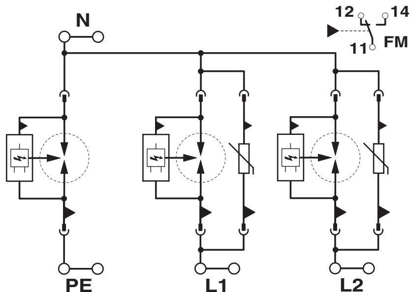
Schaltplan
