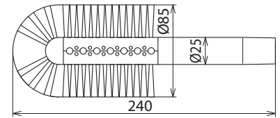
Maßbild STB 85 Z NS
