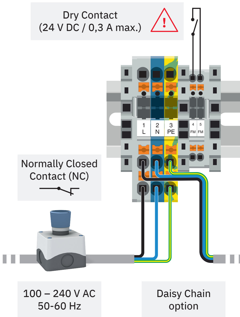
Anschlusszeichnung
