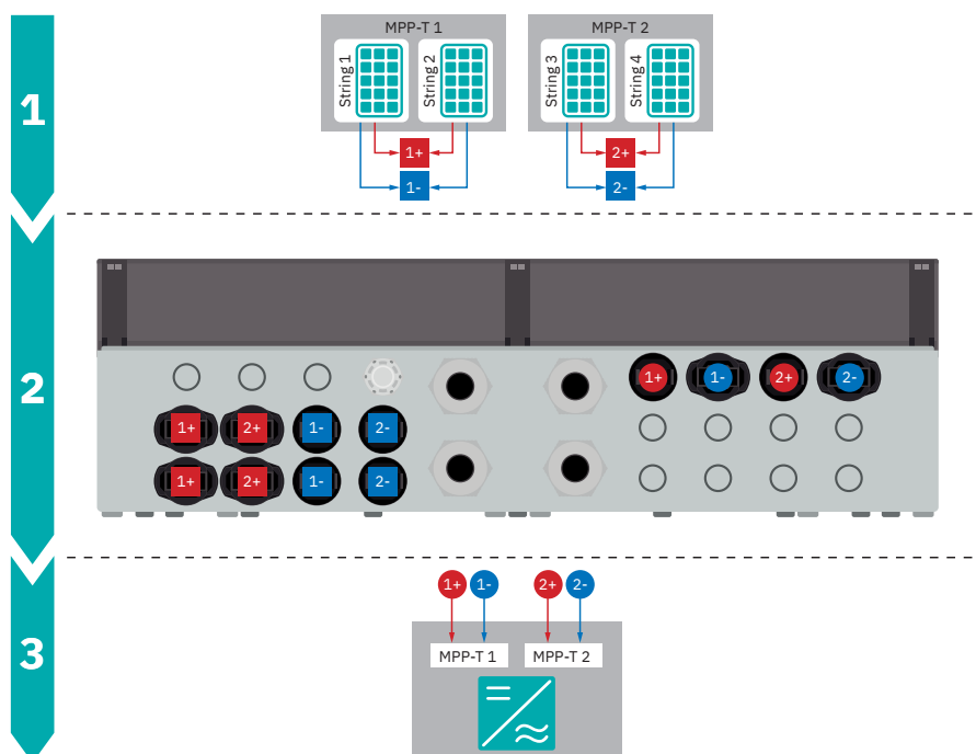
Conexión del string fotovoltaico, así como conexión al inversor
