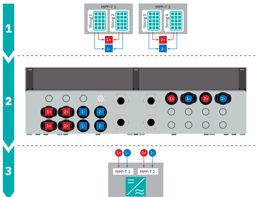
Raccordement des strings photovoltaïques et raccordement à l'onduleur
