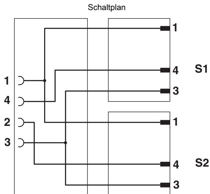
Kontaktbelegung der M12-Buchse und der M8-Stecker
