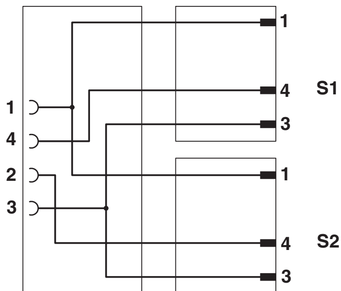
Diagrama eléctrico
