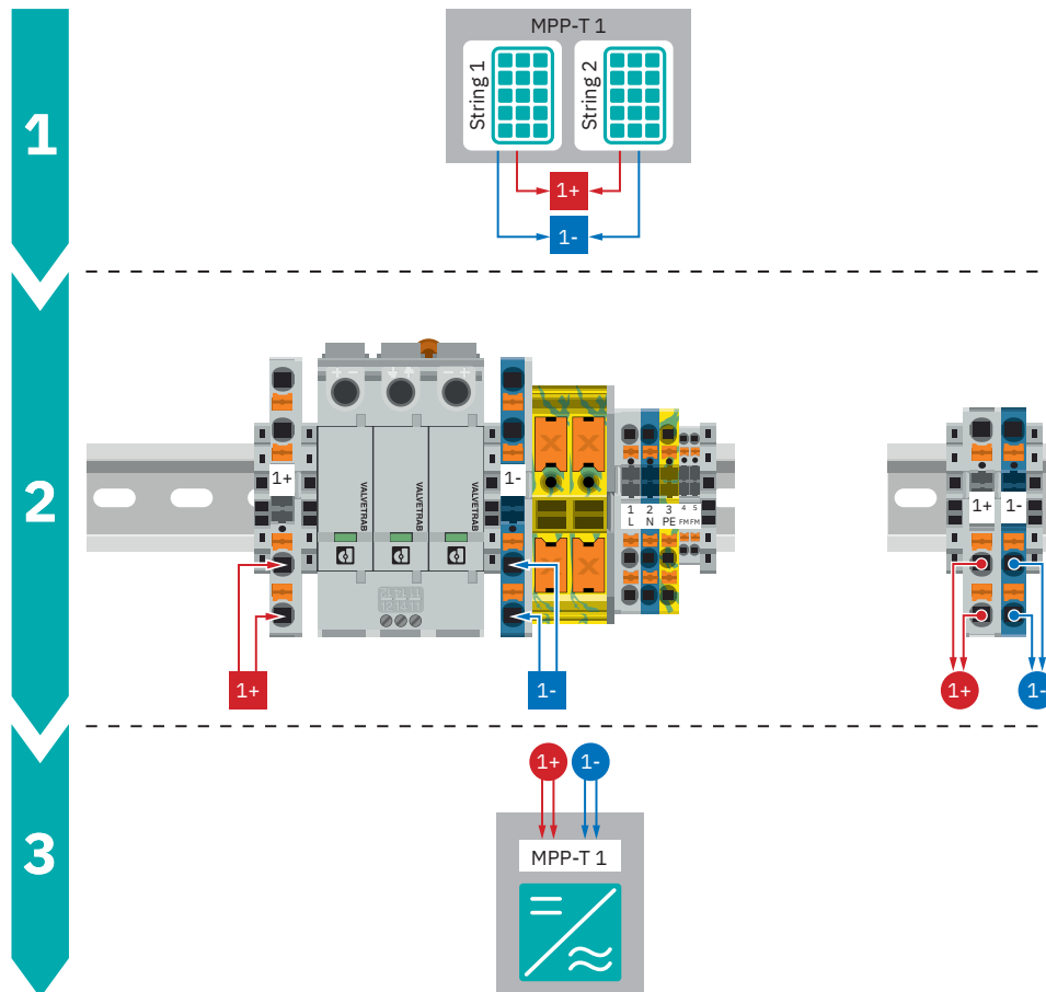
Anschlusszeichnung
