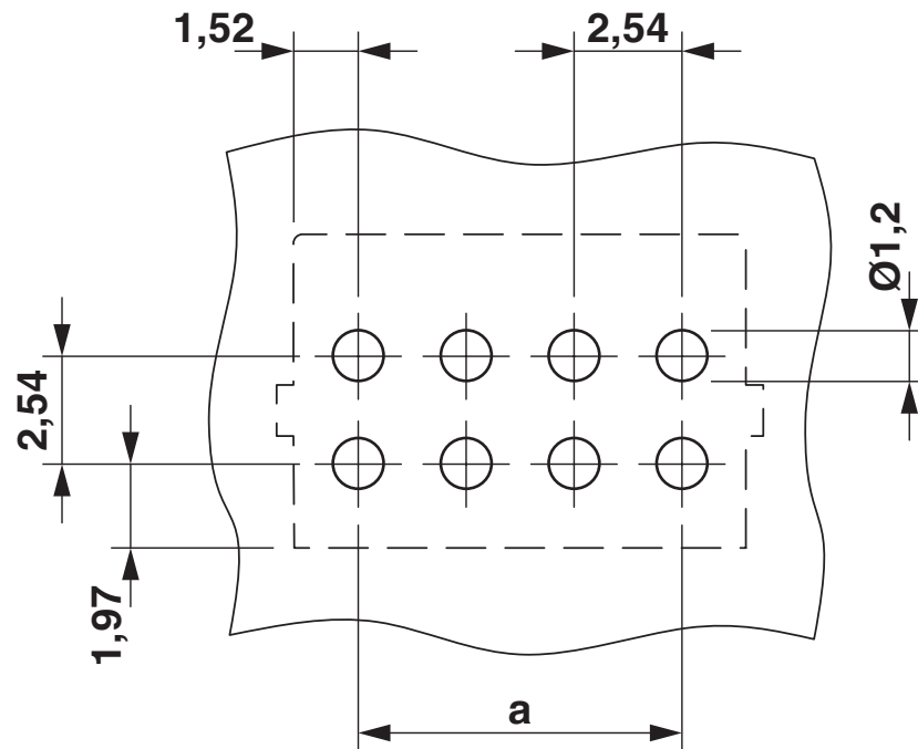
Esquema de taladros/geometría pads soldadura
