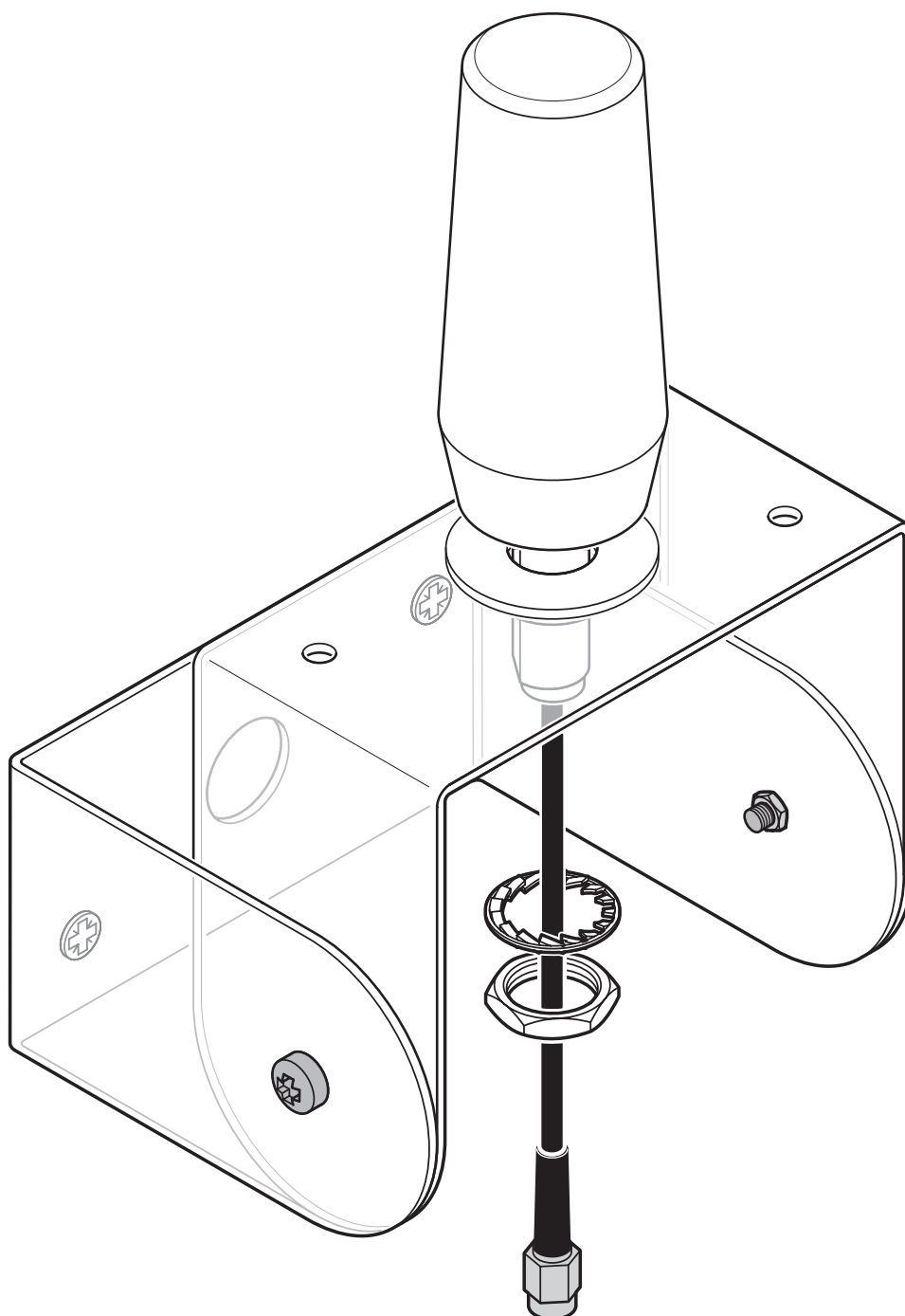
Schemazeichnung
