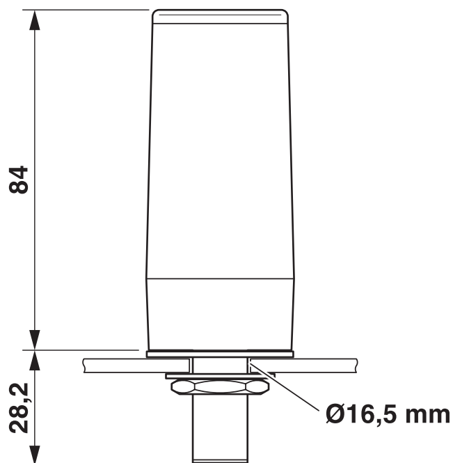
Dessin schématique
