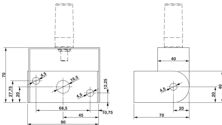
Dessin coté
