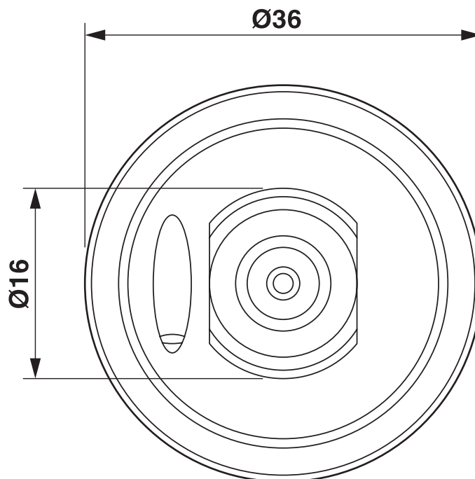
Dessin coté
