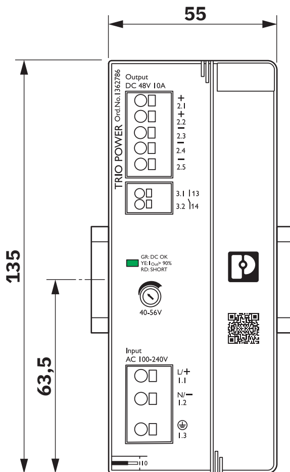
Maßzeichnung
