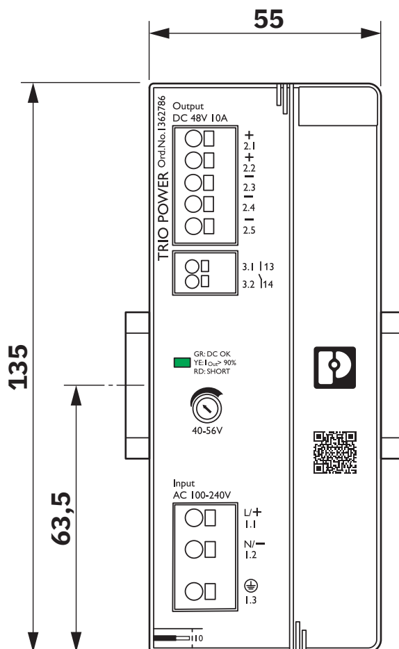
Dessin coté
