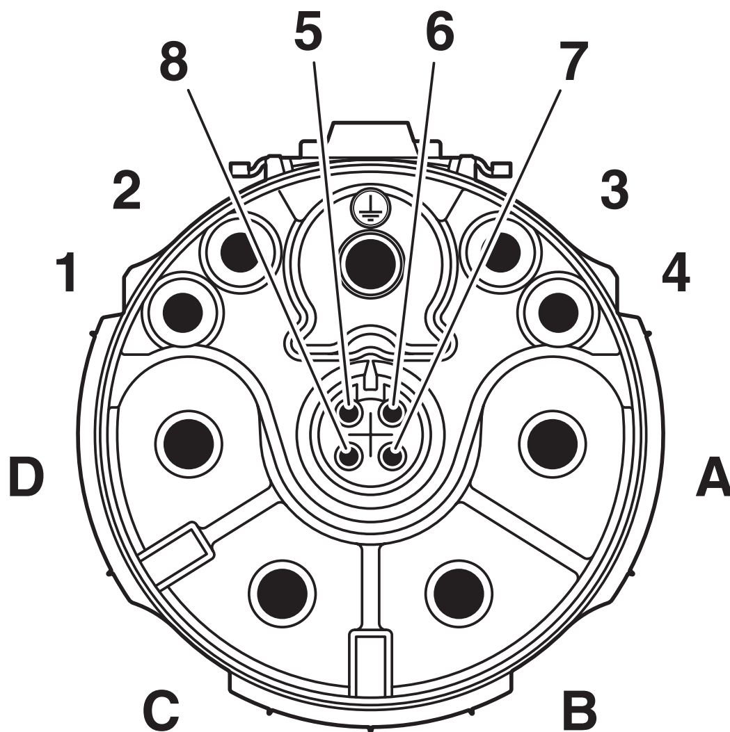
Plano esquemático
