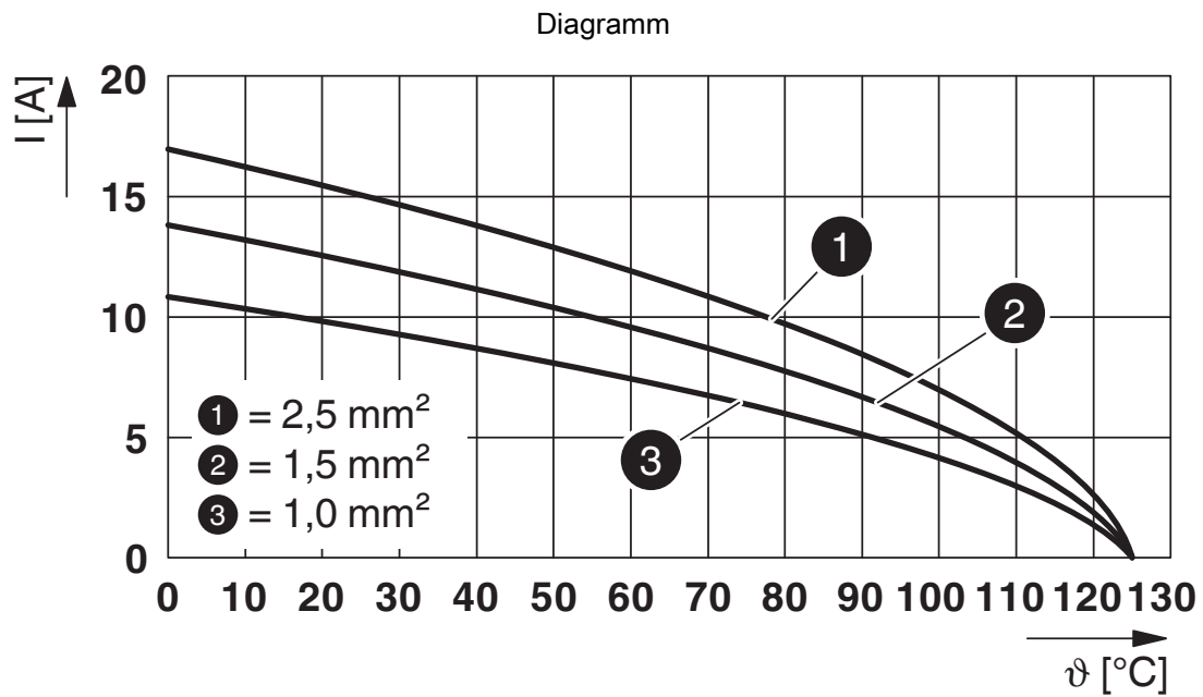
Derating-Diagramm gerollte Kontakte
