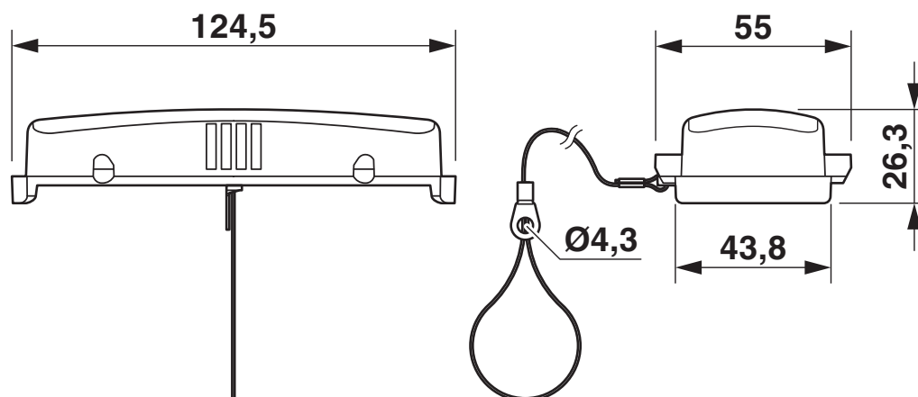
Dessin coté
