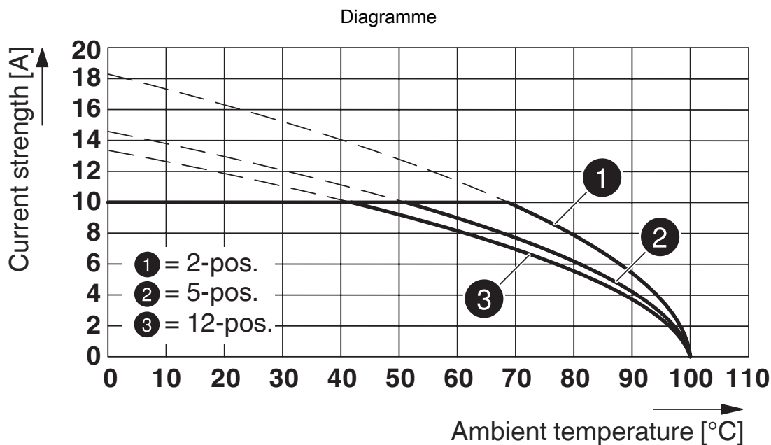
Type : FRONT-MSTB 2,5/...-ST avec MDSTBVA 2,5/...-G
