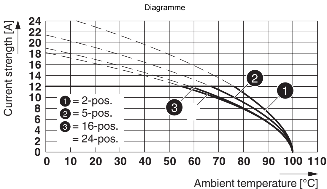
Type : FRONT-MSTB 2,5/...-ST avec SMSTB 2,5/...-G
