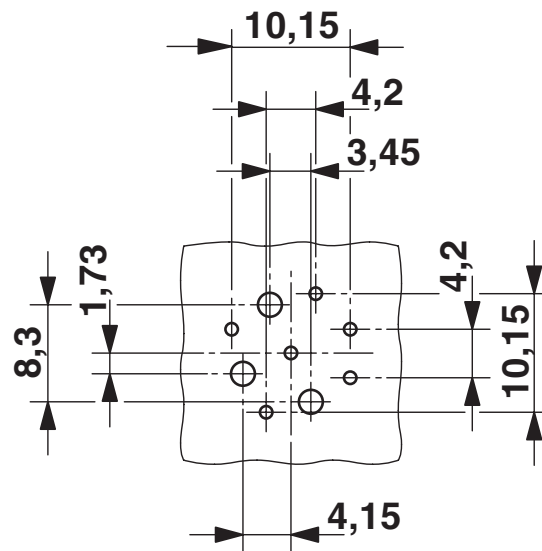
Bohrplan/Lötpadgeometrie
