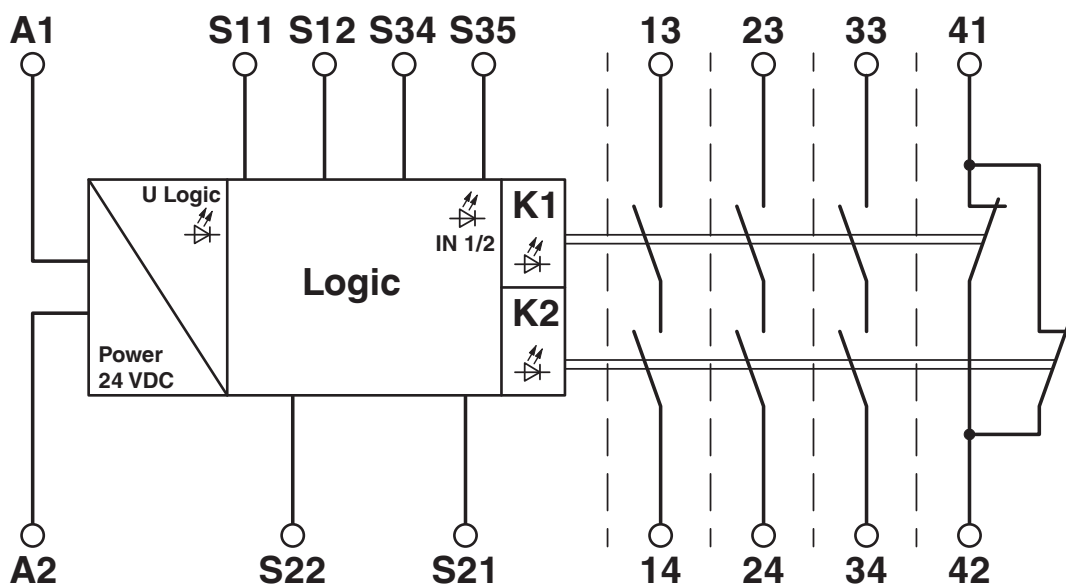
Diagrama eléctrico
