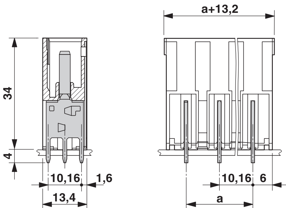
Maßzeichnung
