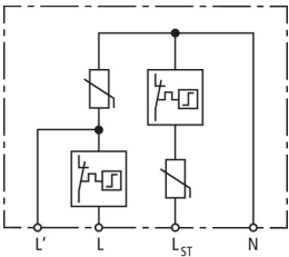
Schema di principio DCOR L 2P SN1864
