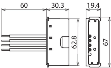
Dimensioni DCOR L 2P SN1864
