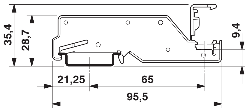
Esquema de dimensiones
