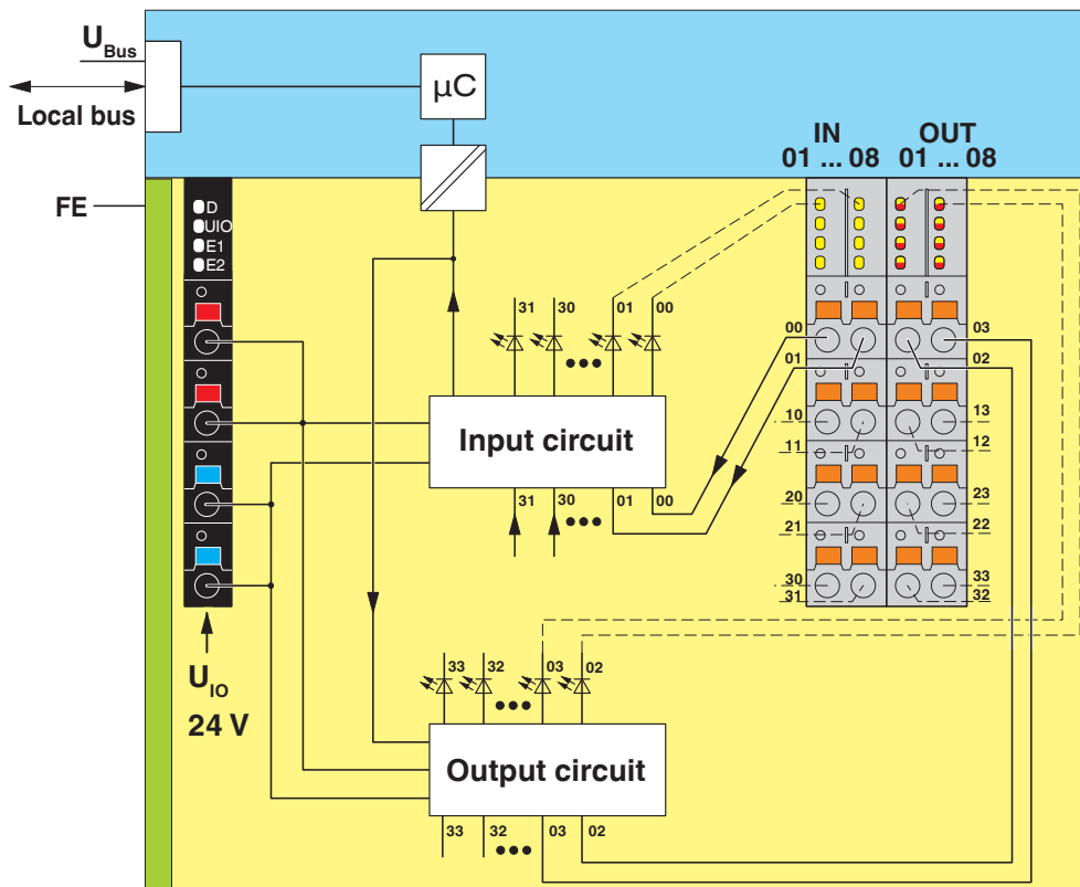
Schéma fonctionnel
