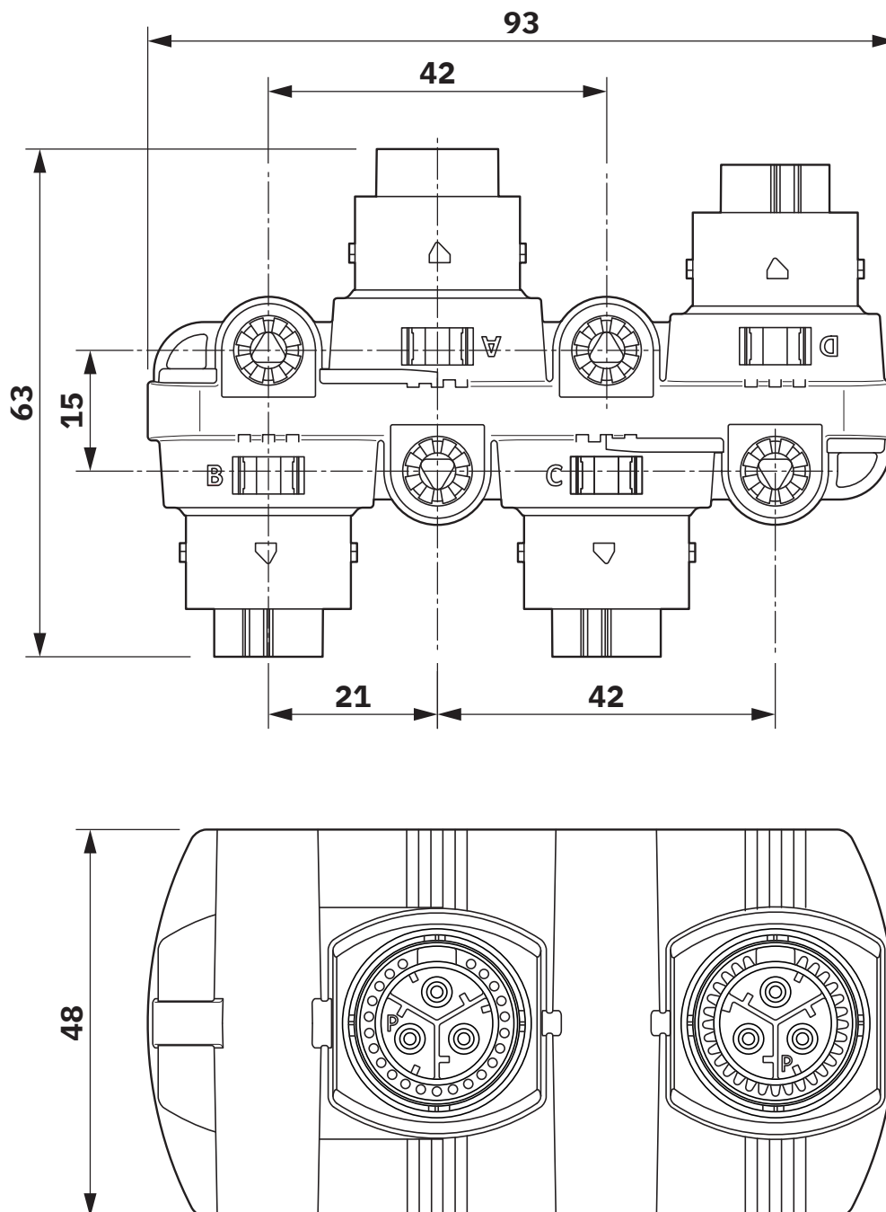
Maßzeichnung
