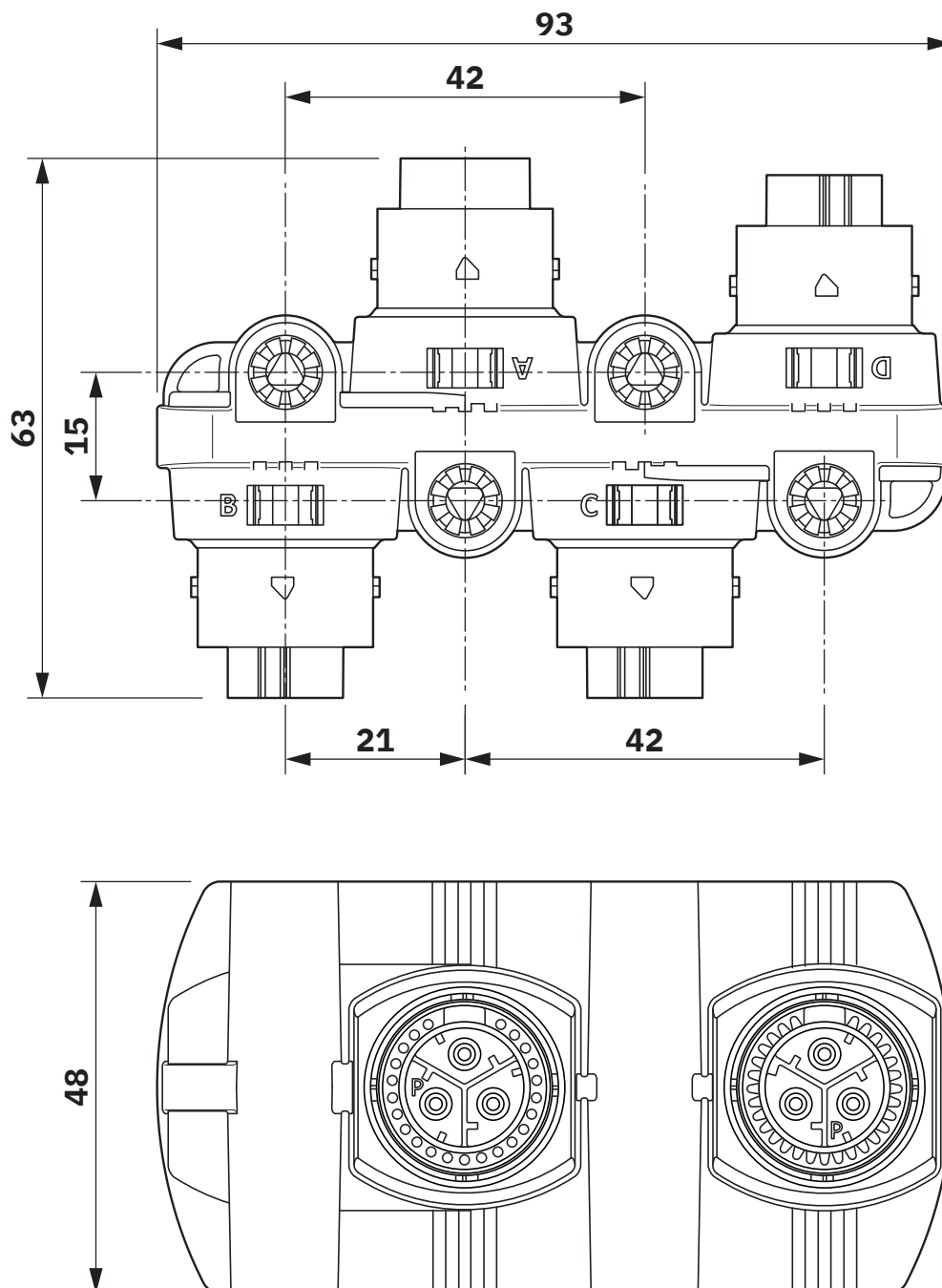
Dessin coté
