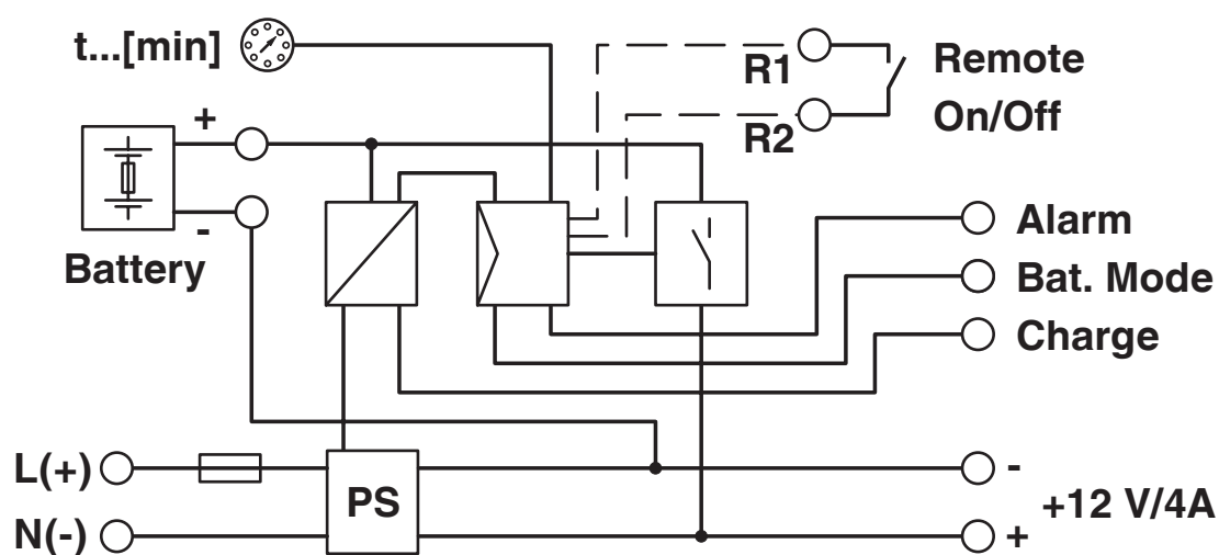
Schéma fonctionnel
