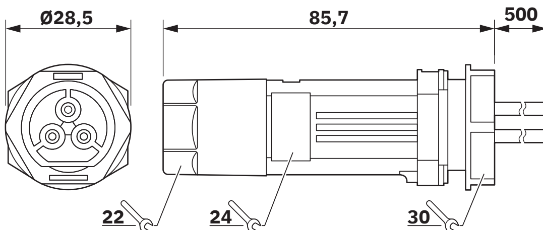
Dessin coté
